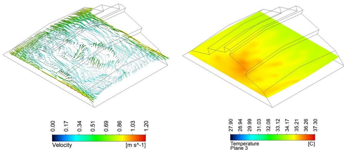
Figura 2. Contornos calculados de velocidad del viento ( \text{m s}^{-1} ) y distribución de temperatura ( ^{\circ}\text{C} ) calculados mediante simulación CFD-3d
